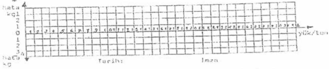
Şekil: 2- Kantar kolu taksimat aralıkları hata çizelgesi
